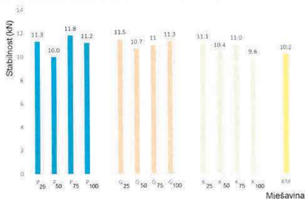
Slika 6. Stabilnost
