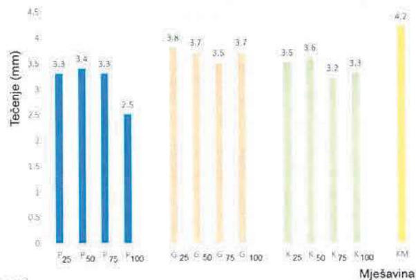
Slika 7. Tečenje
