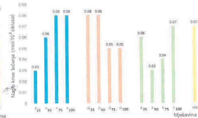
Slika 10. Nagib krive tečenja
