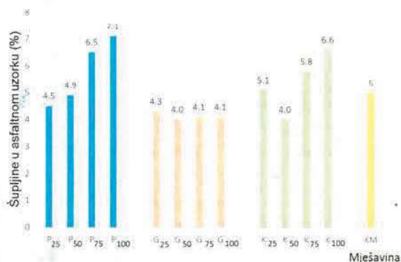
Slika 5. Šupljine u asfaltnom uzorku
