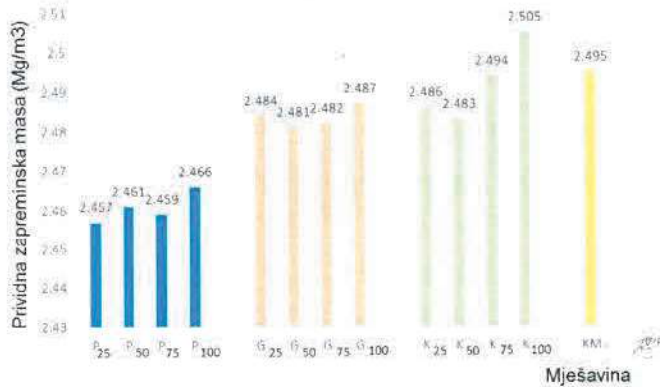
Slika 2. Prividna zapreminska masa
