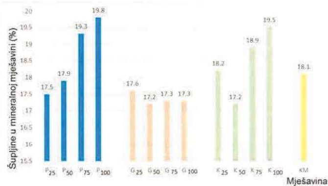
Slika 4. Šupljine u mineralnoj mješavini
