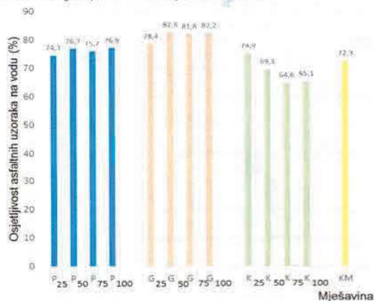
Slika 8. Otpornost asfaltnih uzoraka na vodu
