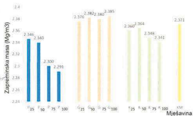
Slika 3. Zapreminska masa
