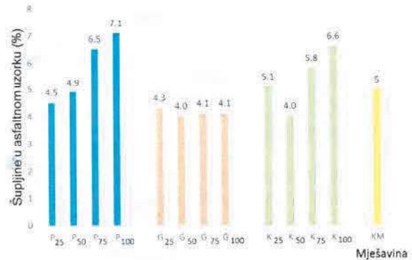
Slika 5. Šupljine u asfaltnom uzorku
