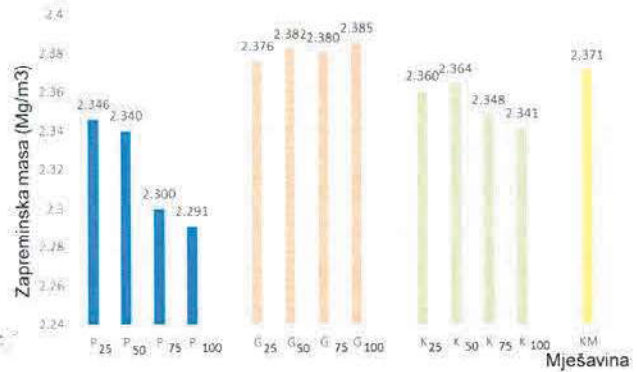
Slika 3. Zapreminska masa
